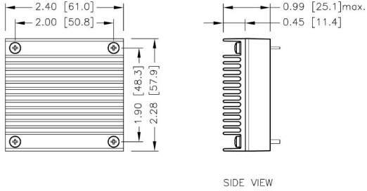
HAE200-□□S□□W -HS 7G-0021A-F
